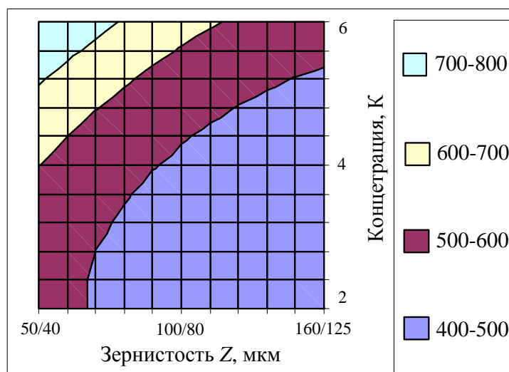
Рис. 3 Двумерные сечения поверхности отклика Q - f(Z, K) : P_H = 1,6 МПа; V = 25 м/с
