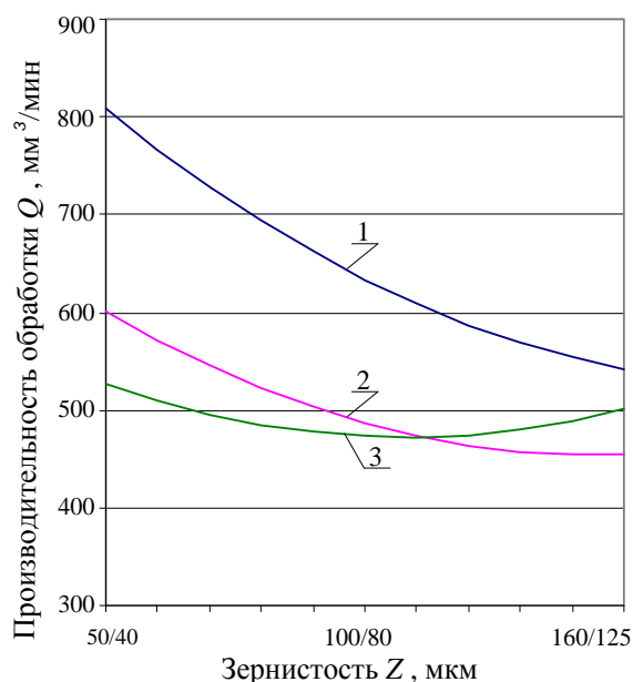
Рис. 4 Влияние Z на Q : P_n = 1,6 МПа, V = 25 м/с;
