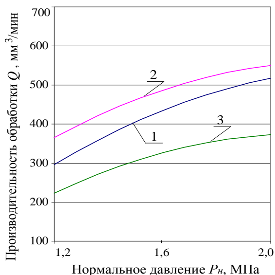
Рис. 1 Двумерное сечение поверхности отклика Q - f(P_n, V) : Z = 100/80 ; K = 4
