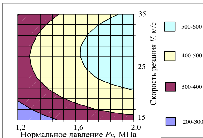
Рис. 1 Двумерное сечение поверхности отклика Q - f(P_n, V) : Z = 100/80 ; K = 4
