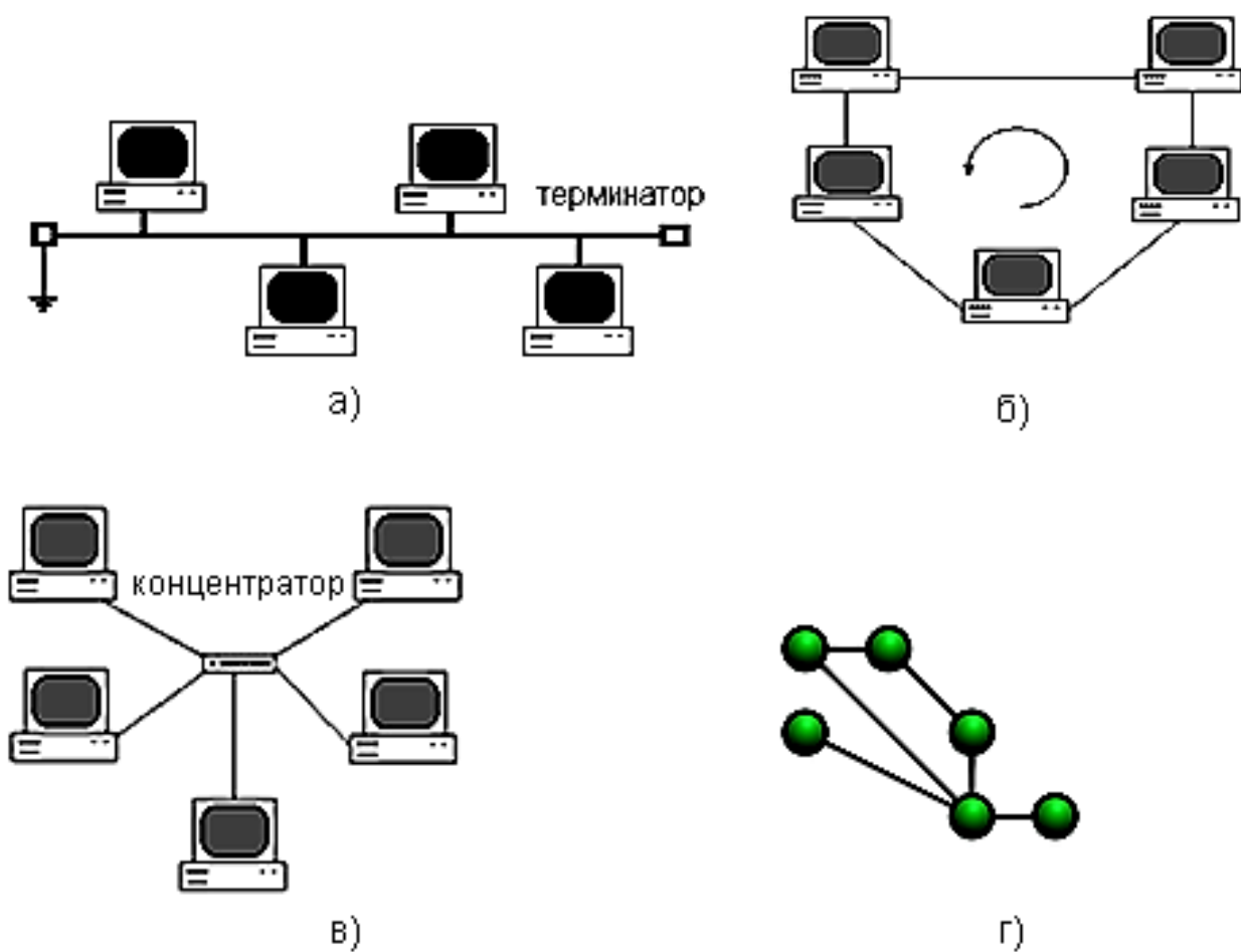
Рис. 5.4. Примеры базовых сетевых топологий
