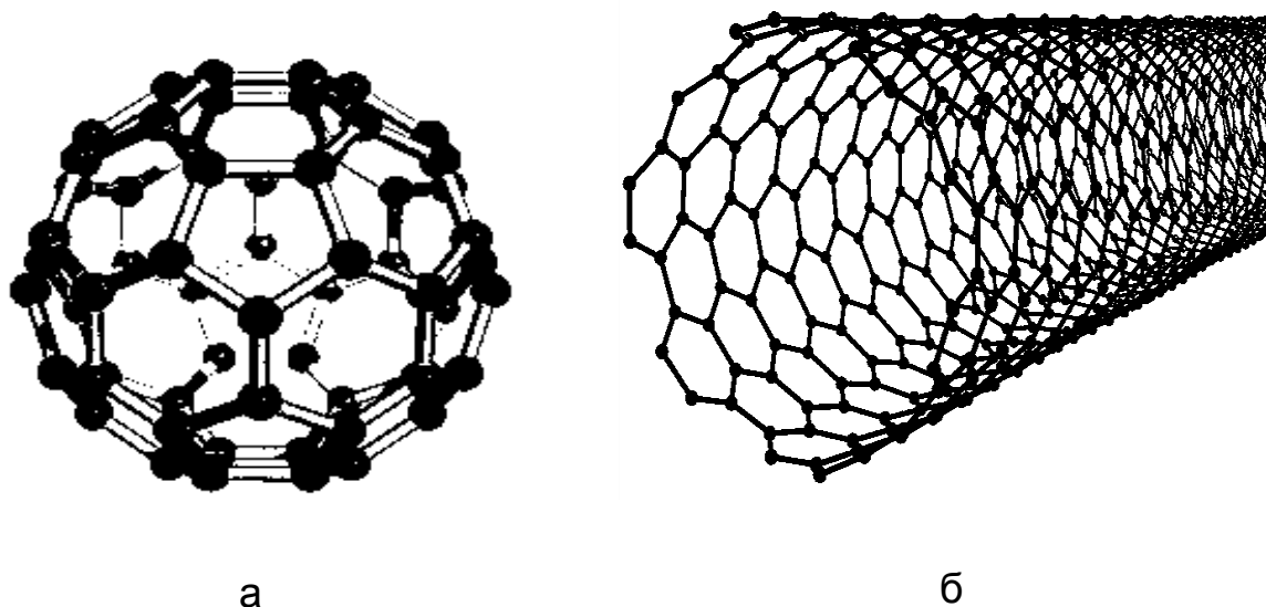
Рис. 4.2. Объемное изображение фуллерена C 60 , как симметричного многогранника с 60 атомами-вершинами (а) и углеродной нанотрубки (б)
