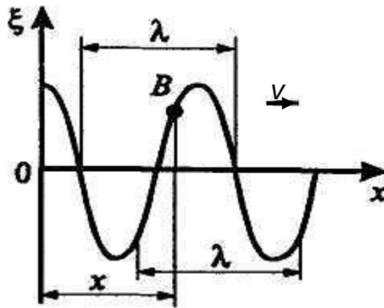
Рис. 3.3. График гармонического колебания (волны)
