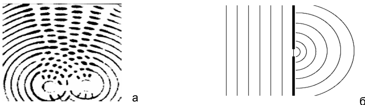
Рис. 3.4. Примеры интерференции двух волн (а) и дифракции плоской волны на отверстии малых размеров (б)
