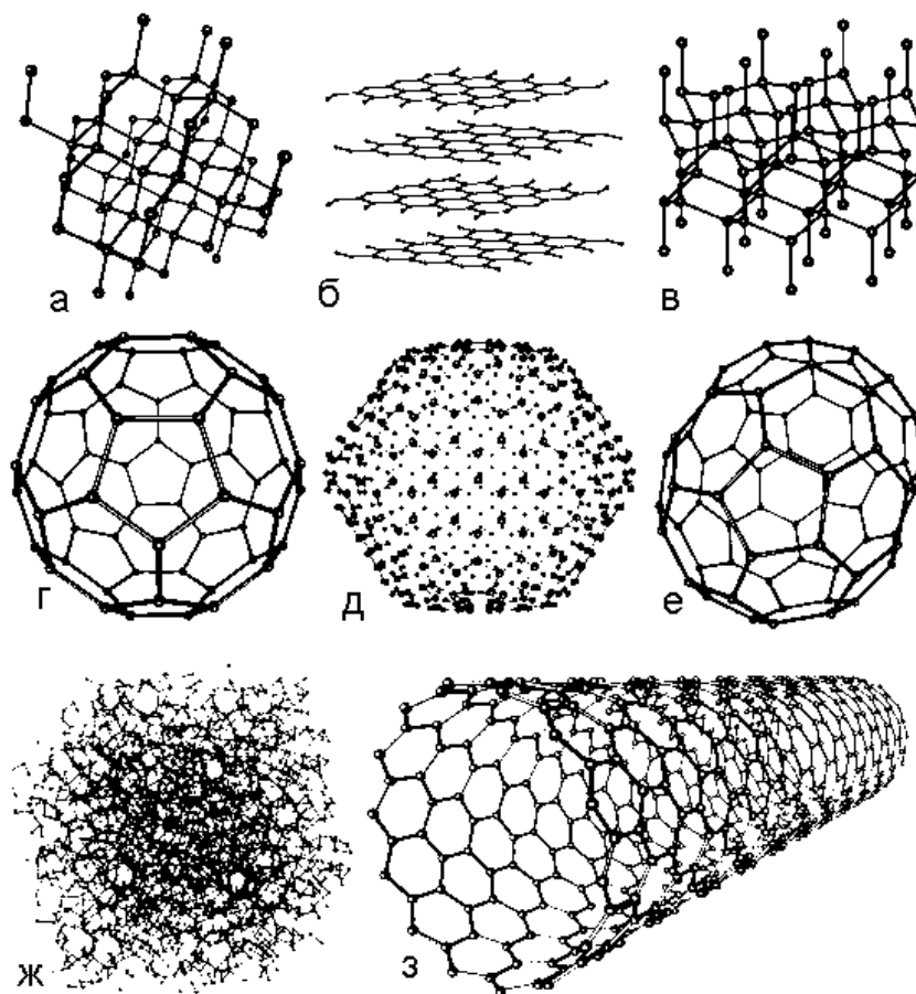
Рис. 4.1. Схемы строения различных модификаций углерода: а – алмаз, б – графит, в – лонсдейлит, г – фуллерен – букибол C_{60} , д – фуллерен C_{540} , е – фуллерен C_{70} , ж – аморфный углерод, з – углеродная нанотрубка
