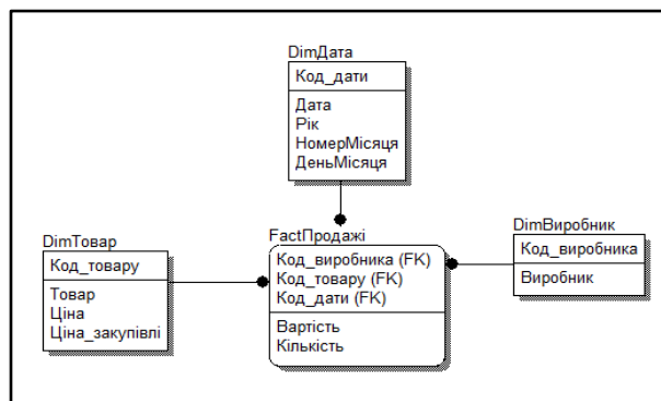
Рис. 2. Схема сховища даних ХлібСД
