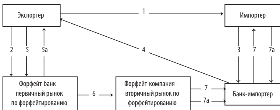
Рис. 11.6. Схема форфейтинга
