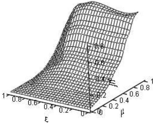
Рис. 2 – Функция расхода РЗ
