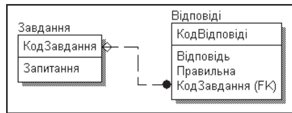
Рис. 1. Схема найпростішої бази даних тестів
