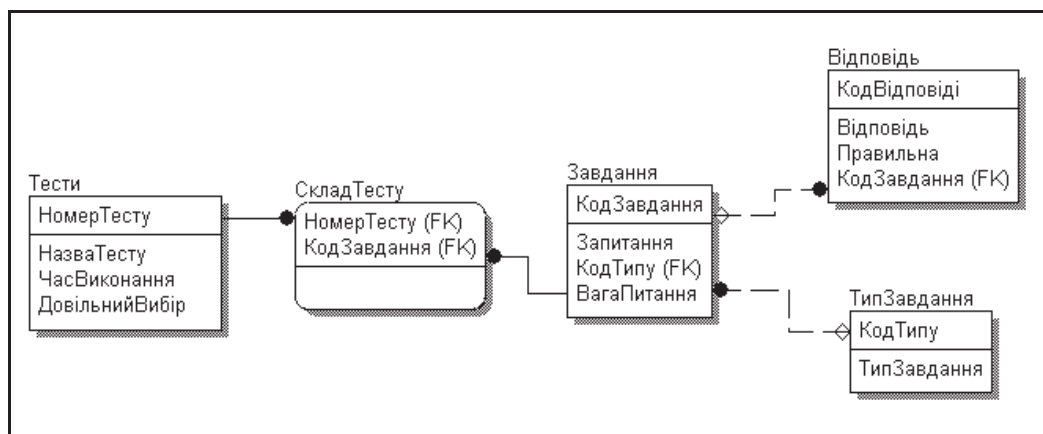
Рис. 7. Схема концептуальної бази даних для реалізації системи тестування
