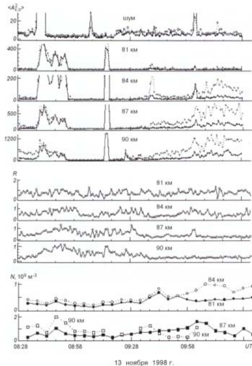
Рис. 5. Высотно-временные вариации \langle A_{o,z}^2 \rangle(z, t) , R(z, t) и N(z, t) , полученные в эксперименте 13.11.1998 г. в период оптической вспышки класса SF
