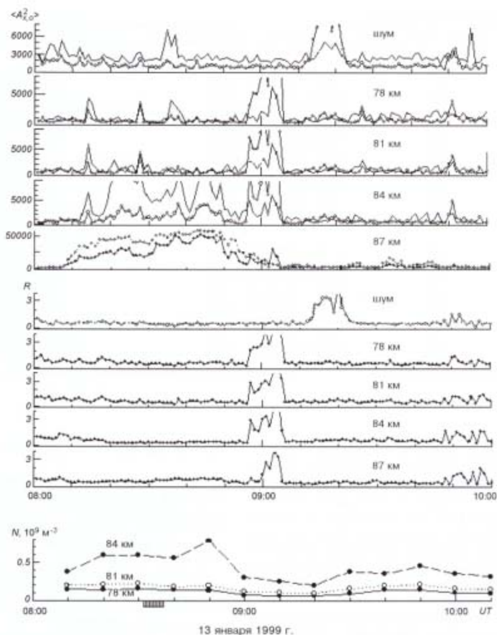
Рис. 1. Высотно-временные вариации \langle A_{\nu, \omega}^2 \rangle(z, t) , R(z, t) и N(z, t) , полученные в эксперименте 13.01.1999 г. в период вспышки рентгеновского излучения класса В4.6. Время вспышки здесь и далее отмечено заштрихованной областью
