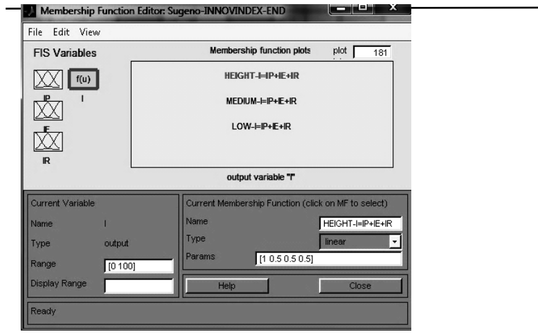
Рис. 5. Установлення лінійної залежності "входів" і "виходу" в Membership Function Editor [Setting the linear relationship between the "inputs" and "output" in the Membership Function Editor]
