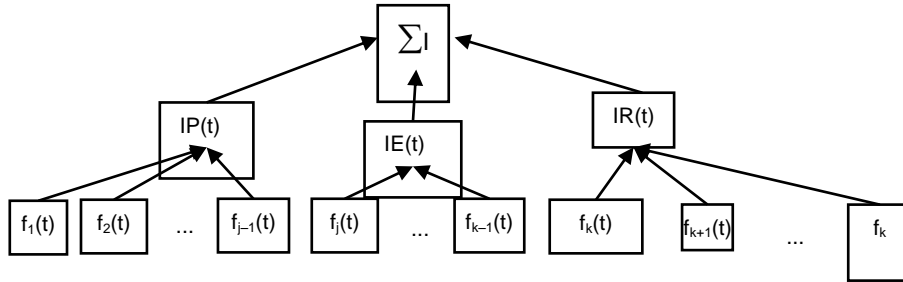
Рис. 1. Ієрархічне дерево логічного висновку [A hierarchical tree of logical deduction]
