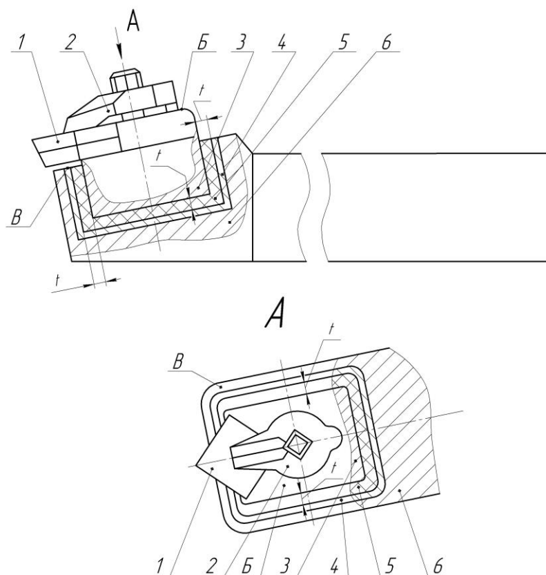
Рис. 1. Общий вид резца.
