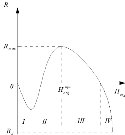
Рис. 2. Очікувана залежність у фазовому просторі \langle R; H_{org} \rangle
