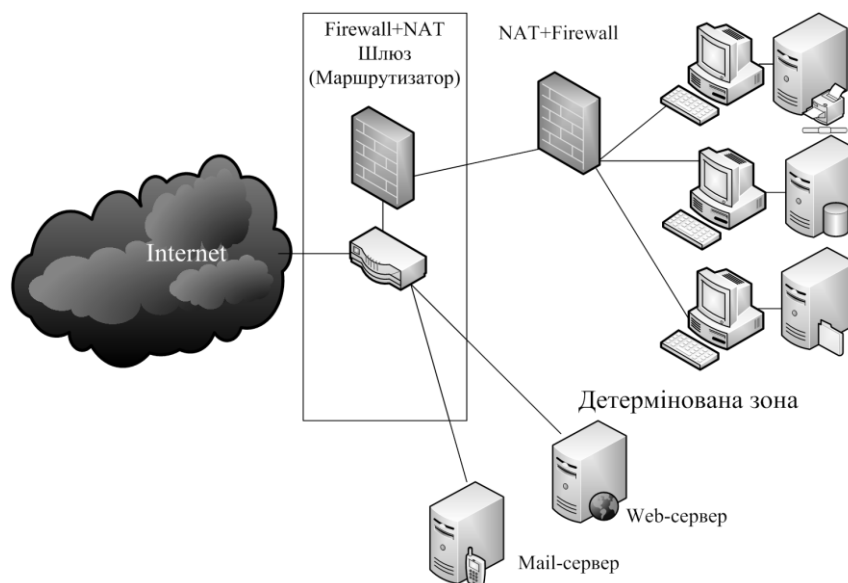
Рис. 2.2. Трансляція фіксованої внутрішньої адреси у фіксовану зовнішню
