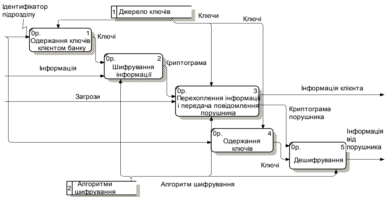
Рис. 1.16. Декомпозиція моделі активної атаки "маскарад"
