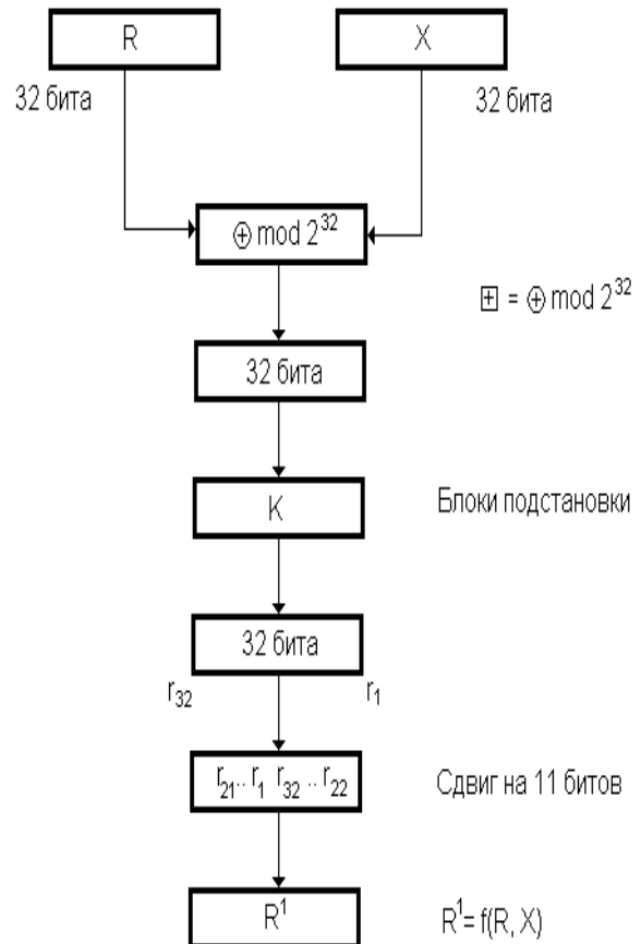
Рис. Б2. Функція перетворення f(R, X) в алгоритмі ДСТУ 28147-89
