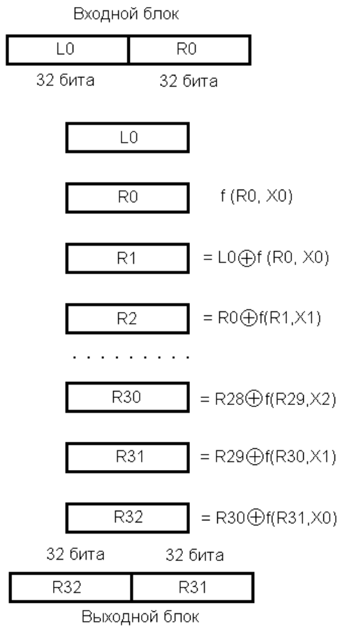
Рис. Б1. Алгоритм шифрування ДСТУ 28147-89 (режим простої заміни)
